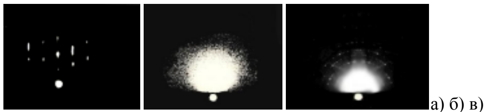
4-расм. CoSi 2 /Si (111) сирт электронограммаси
