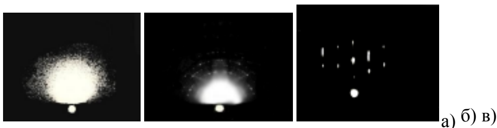
Рис. 4. Электронограммы поверхности CoSi 2 /Si (111)
