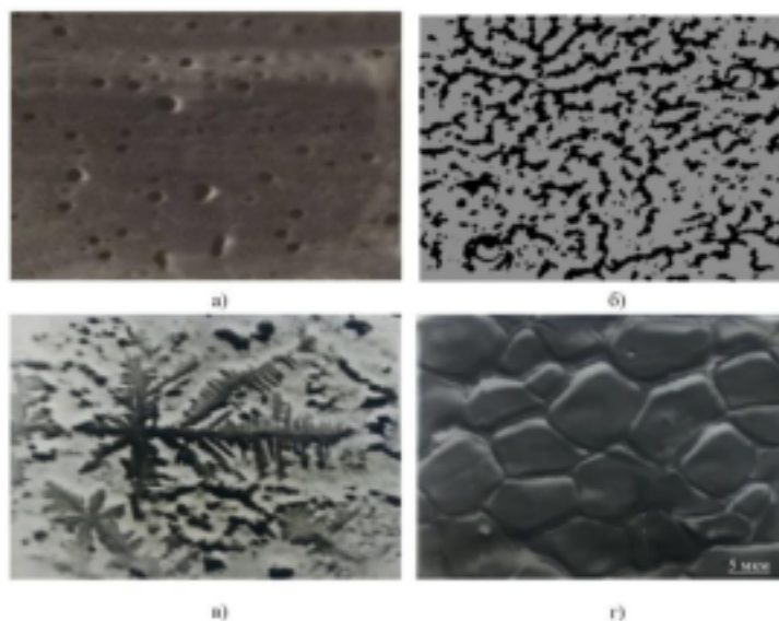
а) 6 \cdot 10^{14} ; б, в) 5 \cdot 10^{15} ; г) 6 \cdot 10^{16}
