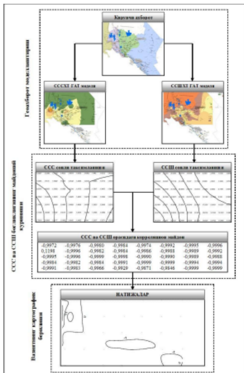
3-расм. «Силжийдиган ойна» усули асосида амалга ошириш алгоритми
