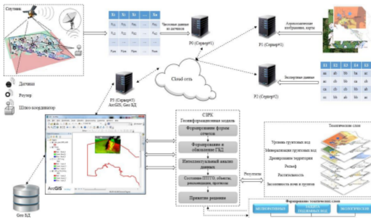
Рис.1. Концептуальная схема обработки всей доступной информации в процессе комплексного исследования ПТГГО
