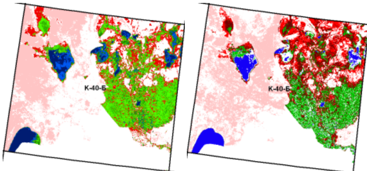
Рис. 2. Растровая классификация на основе космических снимков Таблица 1
