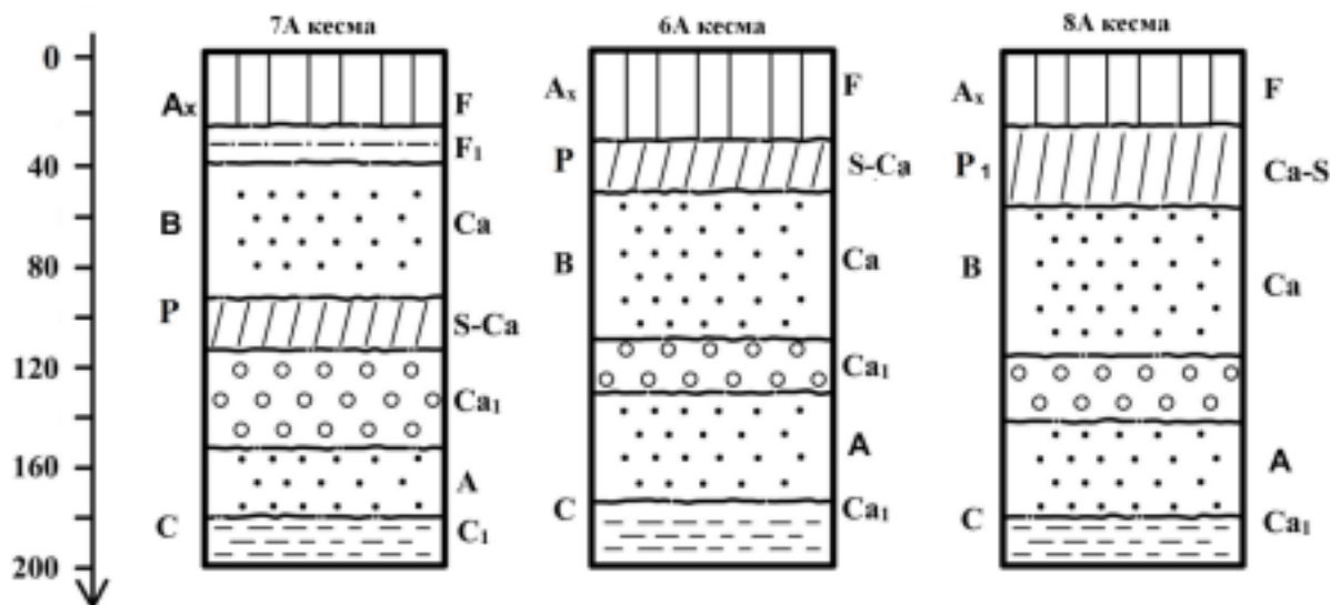
16-расм. Педогеокимёвий барьерни схематик тасвири
