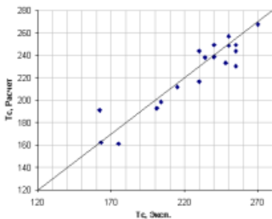
Экспериментальные и рассчитанные значения T_g ( ^{\circ}\text{C} ), для структур контрольной выборки
