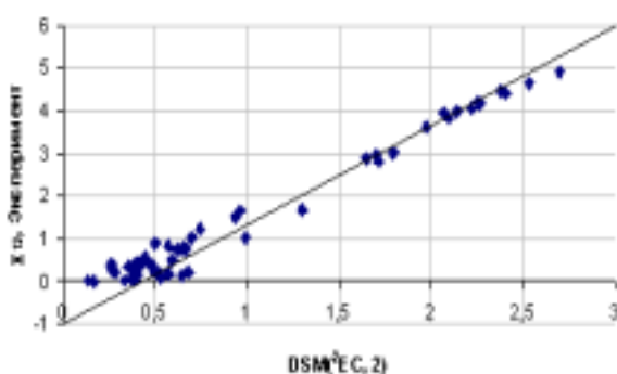
Рис. 3. Зависимость рассчитанных значений DSM^{(2)EC, 2} от экспериментальных значений параметра Флори-Хаггинса для обучающей выборки
