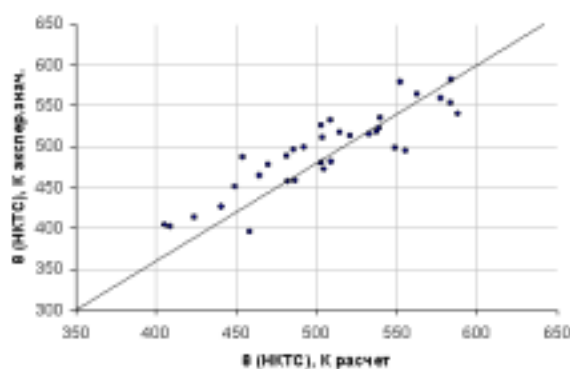
Рис. 5. Зависимость экспериментальных от рассчитанных с использованием значений НКТС, °К дескриптора DMS( EC)
