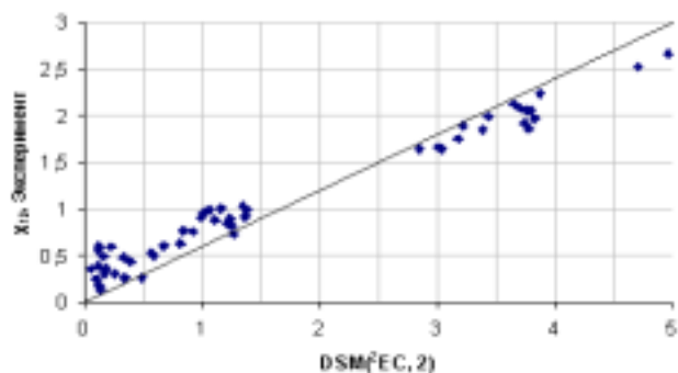
Рис. 4. Зависимость рассчитанных значений DSM^{(2)EC, 2} от экспериментальных значений параметра Флори-Хаггинса для контрольной выборки
