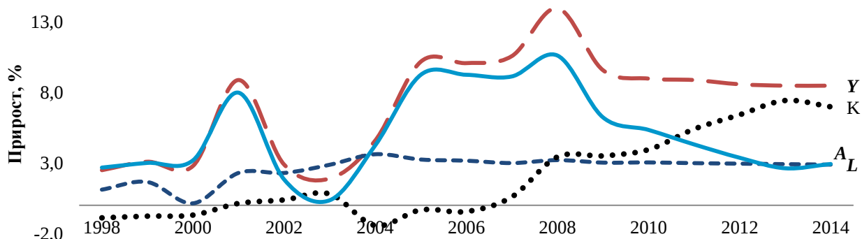
Рис. 2. Параметры производственной функции малого города
